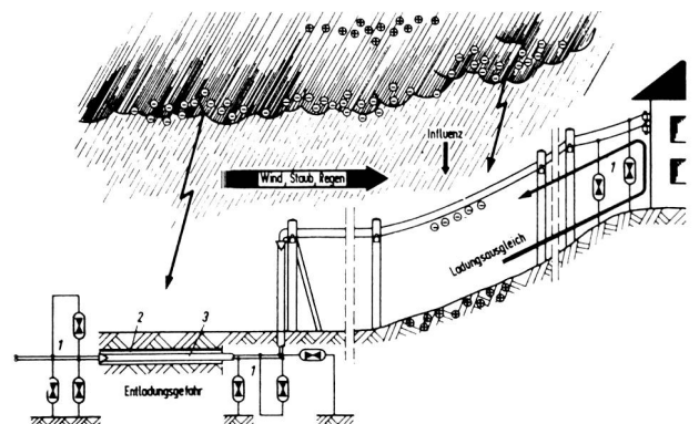
Fig. 2 Äussere Störquellen von Telefonanlagen. Elektro-statische Aufladungen, direkte und indirekte Blitzeintrschläge, eingezeichnet die Lage der Gasentladungs-Überspan-nungsableiter (1) auf Freileitungen und Fernmeldekabeln (2 Kabelschacht, 3 Kabelmantel), (nach Dr. phil. nat. Gustav Puri, Rapperswil, Leiter der techn. Abt. R der Cerberus AG Männedorf).
