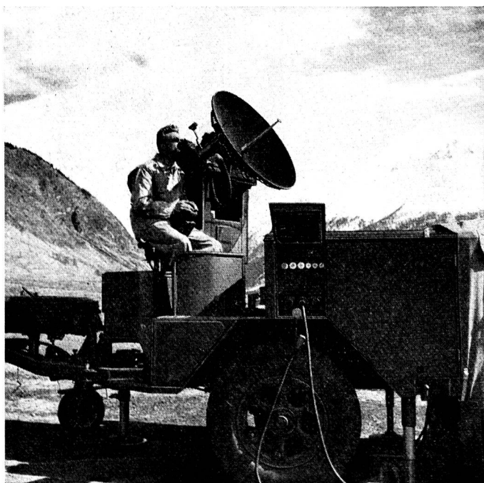
Feuerleitgerät «Fledermaus» mit ALBIS Feuerleitradar AFR 50
