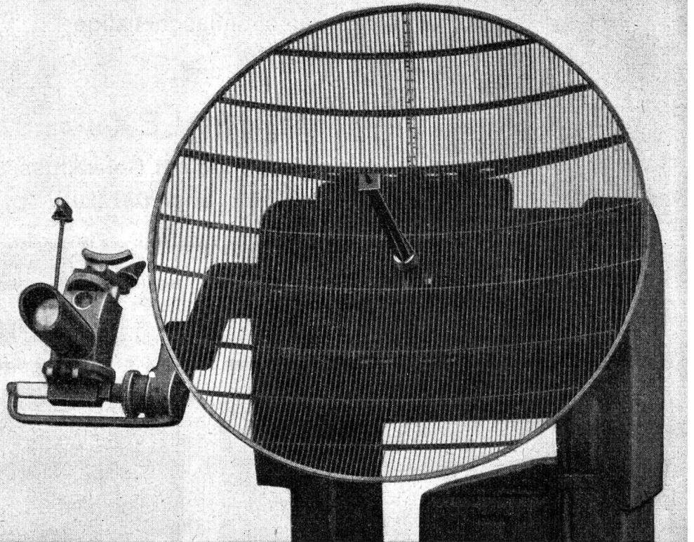
ALBIS-Parabol-Antenne für Suchen und Folgen
