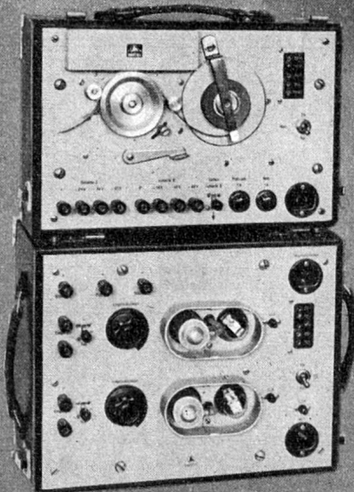
Impulsschreiber mit Zusatzgerät zur graphischen Aufnahme der Oeffnungs- und Schliessungszeiten von Kontakten.
