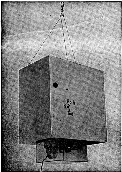
Radio-Sonde (Messgeräte und Sender)
