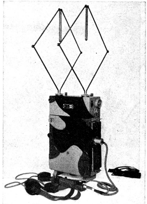
Tragbares Gerät für drahtlose Telephonie mit Dezimeterwellen
