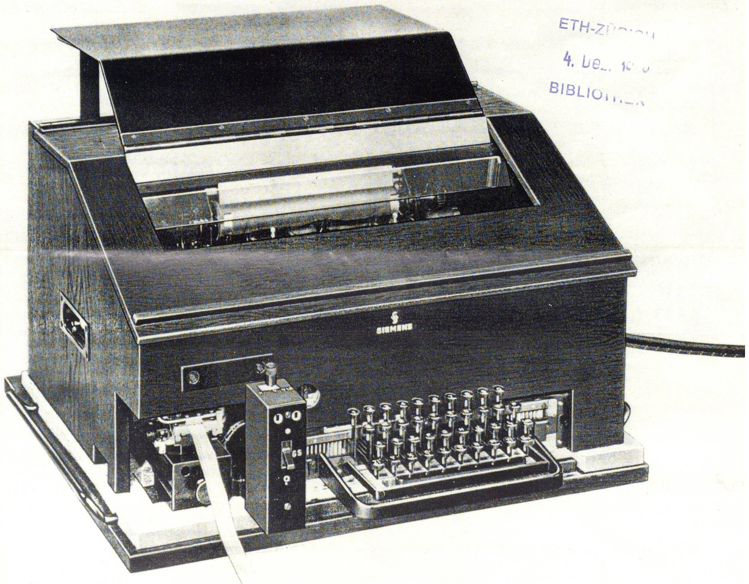
Schlüsselfernschreibmaschine T43. Ausführung: Mechanischer Fernschreiber T, Typ 371 (Blattschreiber), mit Schlüssel-Lochstreifen-Zusatz, Abfühl-,Vorschub- und Stanzeinrichtung links. (Foto: Siemens & Halske 1944)
