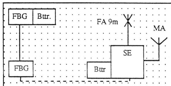
SE-225/t1 (Version portable avec FBA)
