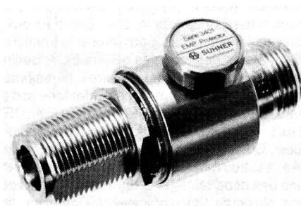
RF-dichte Durchführung mit integriertem NEMP-Ableiter
