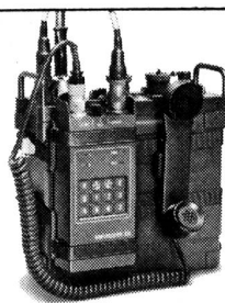
Sprachchiffriergerät GRETACODER 210
