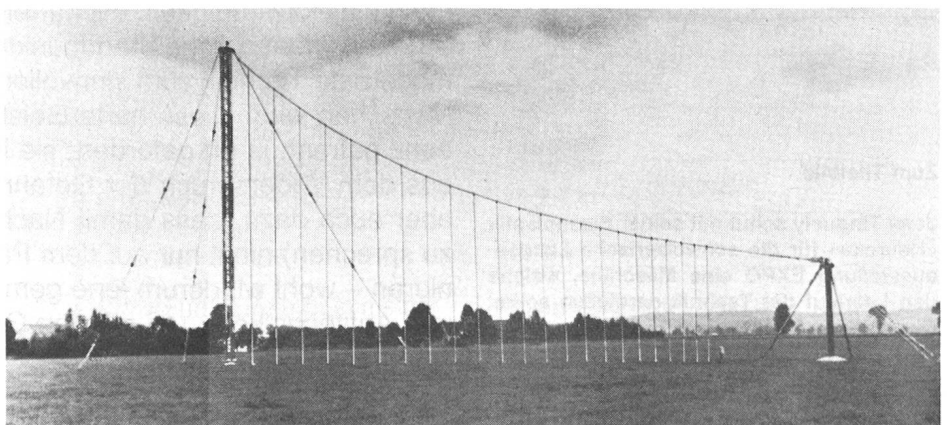
Empfangsantenne zur Elektronischen Aufklärung im Kurzwellenbereich. Damit ist die Elektronische Aufklärung (EA) über Grenzen hinweg möglich.
