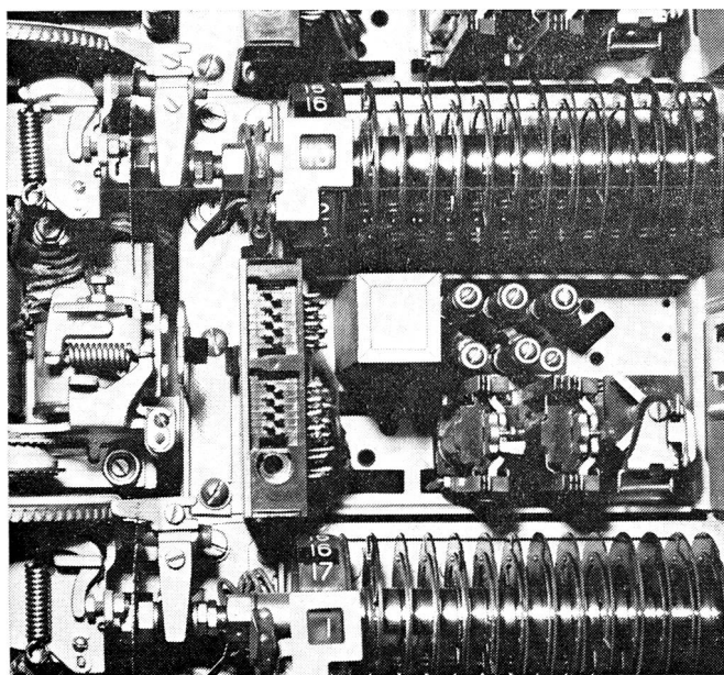
7-A Folgeschalter
