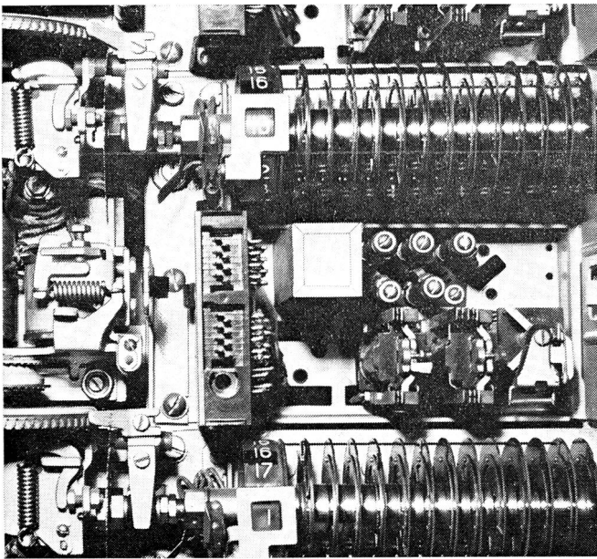
7-A Folgeschalter
