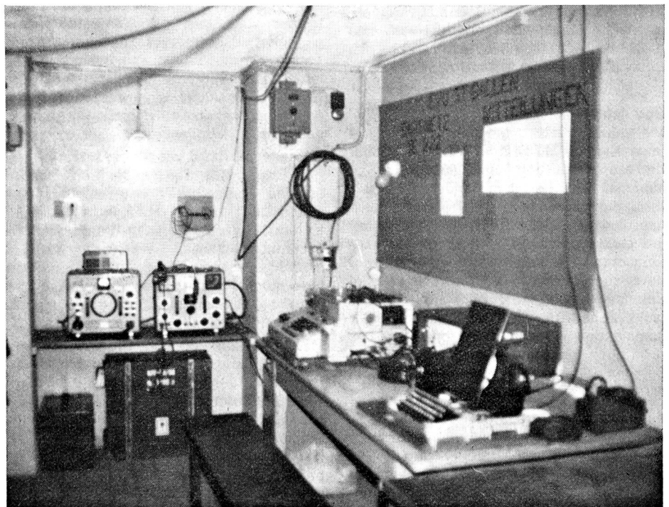
Blick in unser Funklokal mit betriebsbereiter Funkstation SE-222/KFF
