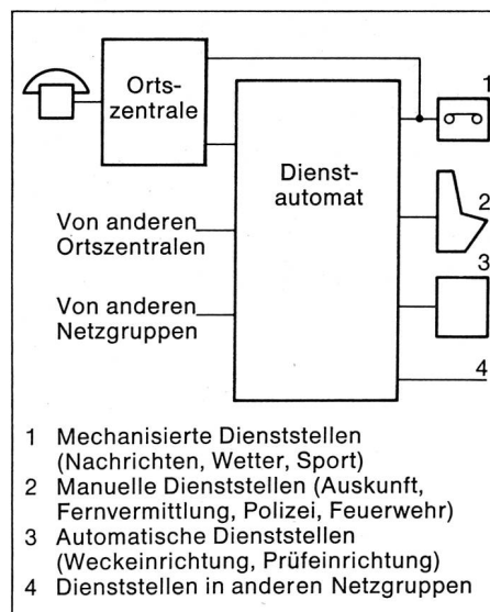
Prinzip des Dienstautomaten für dreistellige Dienstnummern
