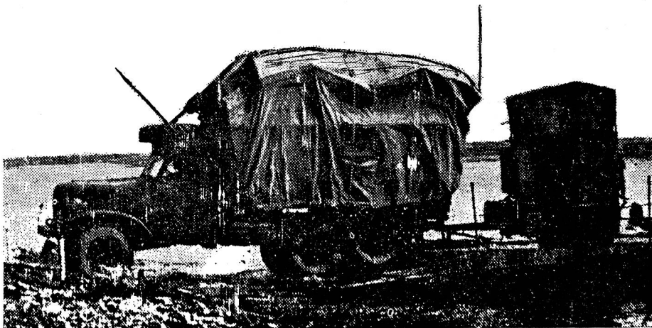
Funkmess-Station der Truppenluftabwehr auf dem Marsch. Im Zweiradanhängen befindet sich das Reservestromaggregat. Die Antennenanlage ist abgeklappt auf dem Dach des Stationsfahrzeuges gelagert.
