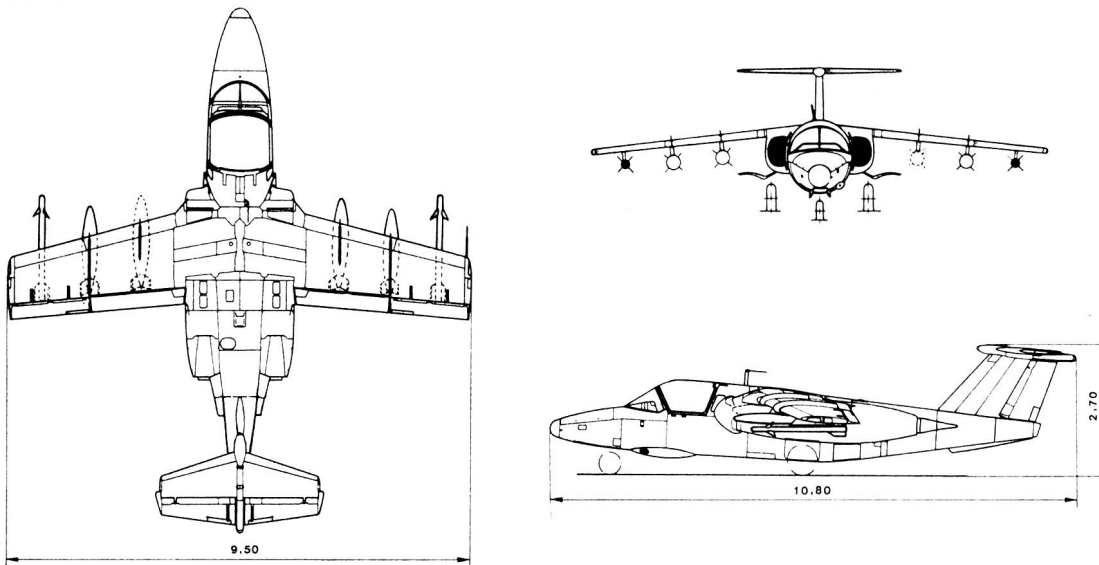
Saab-105
