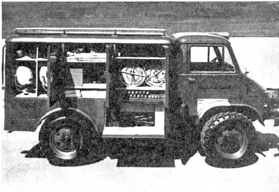
UNIMOG-S als Pionierfahrzeug
