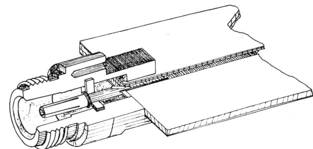
Übergang Koaxialleitung — Triplate
