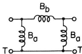
Äquivalenter Kreis für Mittelliniendarstellung
