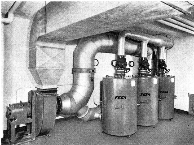
Ventilationsraum einer Sanitätshilfsstelle mit 3 Gasfiltern von je 600 m 3 /h, das heisst 1800 m 3 /h bei Gasfilterbetrieb und 5400 m 3 /h bei Frischluftbetrieb.
