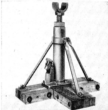
Mechanisch und hydraulisch
