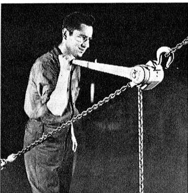
PULLER Rätchenflaschenzüge
