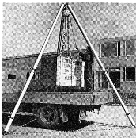
Dreibeine HERCULES
