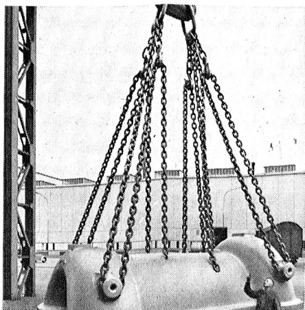
HERC-ALLOY legierte Ketten
