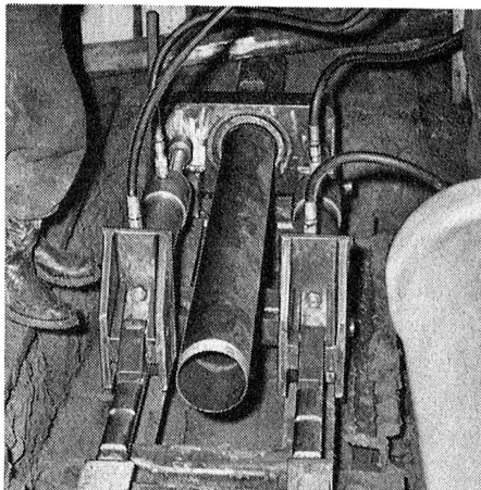
Röhrenstosspressen mech. und hydr.
