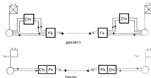
Abb. 8: Alte und neue Verfahren der Uebermittlungstarnung
