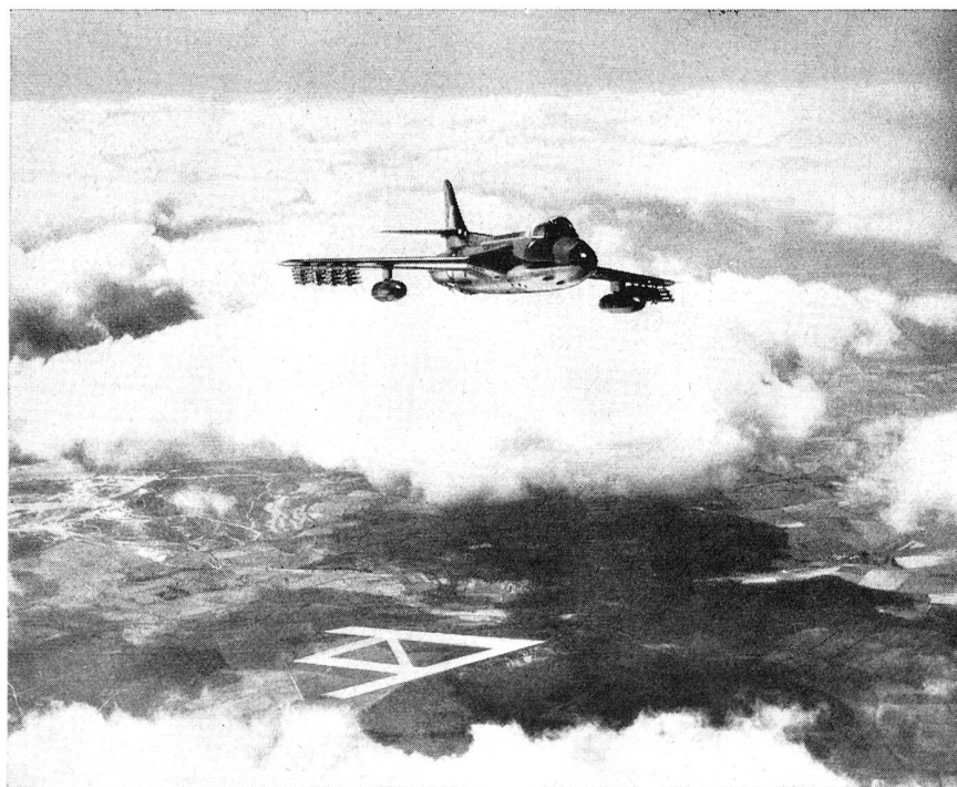
Wirkungsvoller Erdkampfeinsatz mit Flugzeugraketen HISPANO SUIZA «SURA» Feststoffrakete, Kaliber 80 mm, mit Spreng- oder Hohlladung, für alle Aufhängungssysteme.
