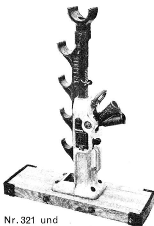
Links: «Meili» Konsol- Wandwinden mit rückschlagfreier Sicherheitskurbel
