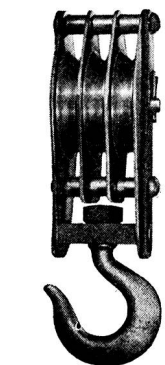
«Meili» Hanfseilflaschen No. 1—4
