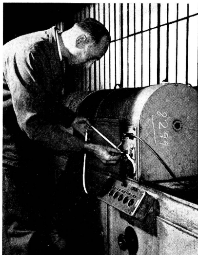
Das Isolieren von Telefon-Montierungsdrähten und Adern von Telefonkabeln erfolgt teilweise in zwei bis drei Farben. Der blanke oder verzinnte Kupferdraht dreht sich mit gleichmässiger Geschwindigkeit und wird gleichzeitig an den stillstehenden Spritzdrüsen vorbeigeführt, so dass eine spiralförmige Markierung entsteht. Durch das Aufspritzen der Masse in warmem Zustand wird erreicht, dass die verschieden gefärbten Kunststoffmassen an den Grenzlinien gut abbinden. Gleichzeitig mit dem Umspritzen wird der Leiter elektrisch geprüft, wobei eventuelle Fehler automatisch auf einem Papierstreifen registriert werden.
