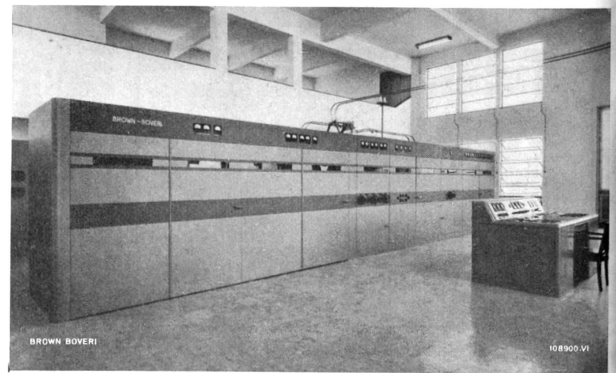
▲ Brown Boveri 100-kW-Kurzwellensender in der Station Rio de Janeiro der Radio- gesellschaft Tupi, Brasilien
