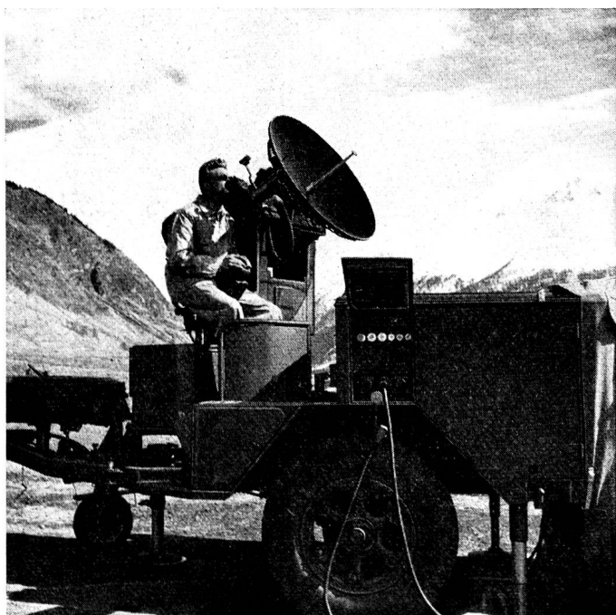
Feuerleitgerät «Fledermaus» mit ALBIS Feuerleitradar AFR 50
