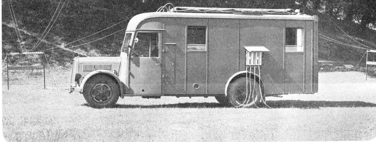
Einer der von uns projektierten und ausgerüsteten Zentralenwagen.
