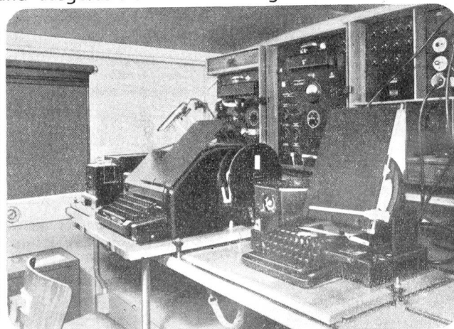
Fernschreibstation mit automatischem Sender und Lochstreifenstanzer für Doppelstrom- oder Eintonübertragung.
