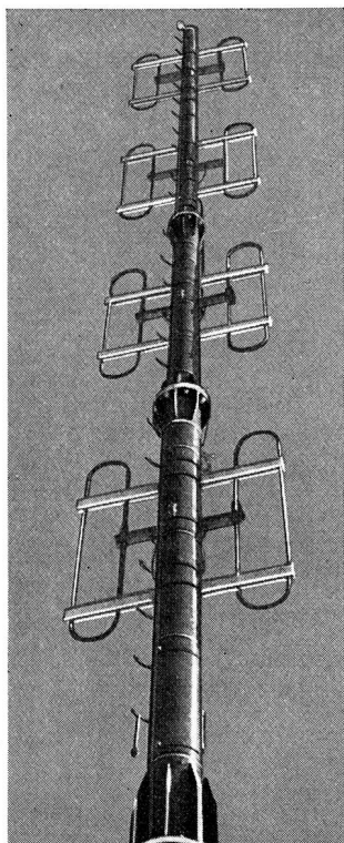
ROHDE-&SCHWARZ Rundstrahler für Autoruf
