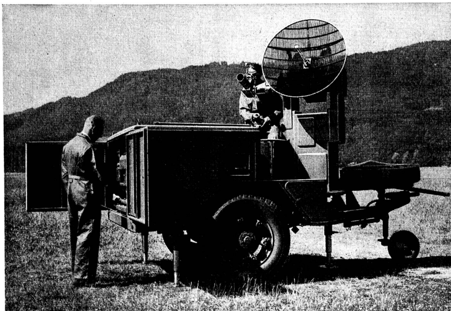
ALBIS-Feuerleitradar AFR 406
