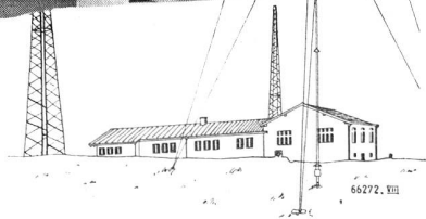
Brown Boveri Sender für den Flugsicherungsdienst in der Sendestation Walköten bei Zürich
