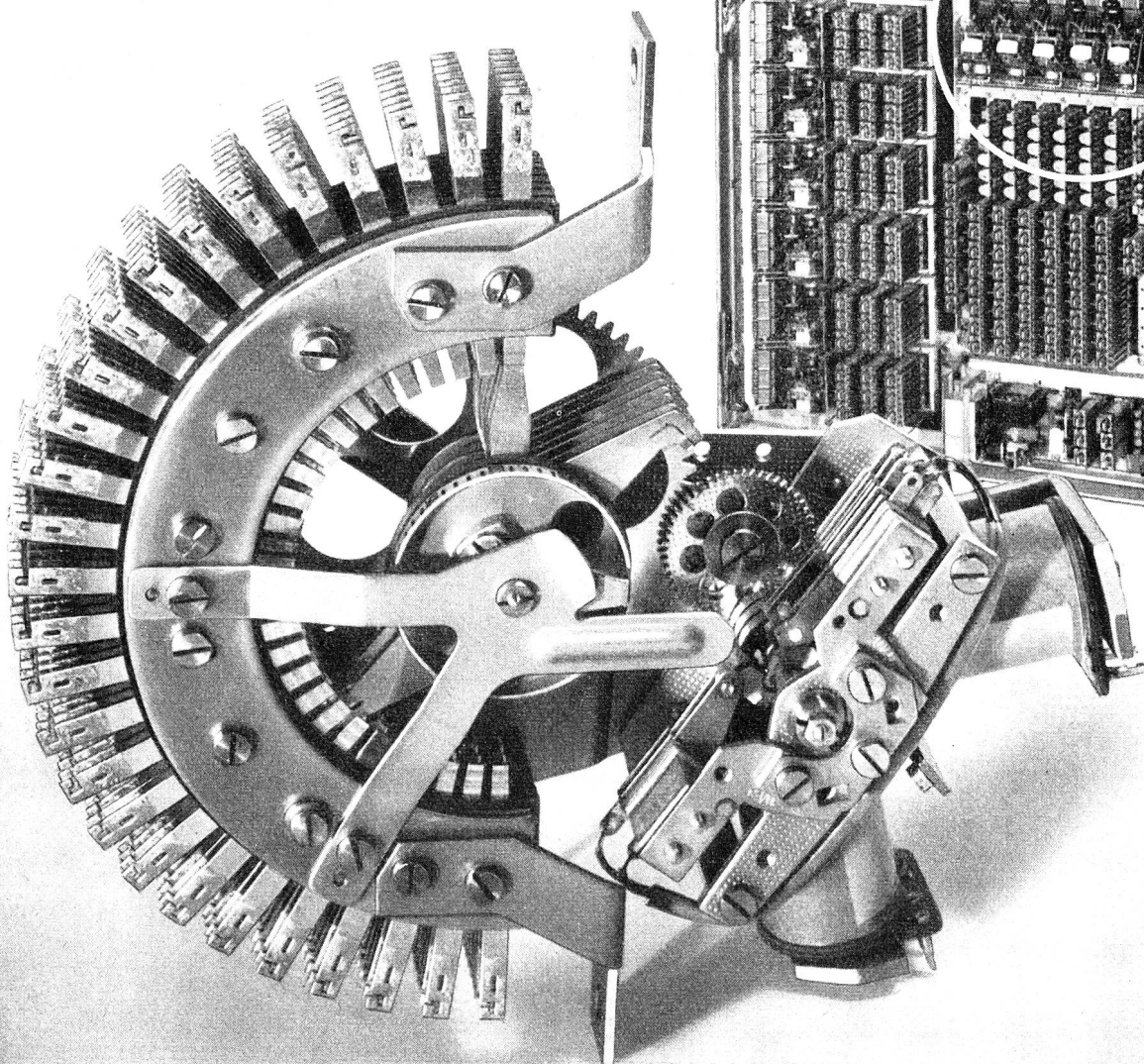
Motorwähler als Anrufsucher in der Haus-Telephonzentrale V/45, für 5 Amtsleitungen und 45 Teilnehmeranschlüsse
