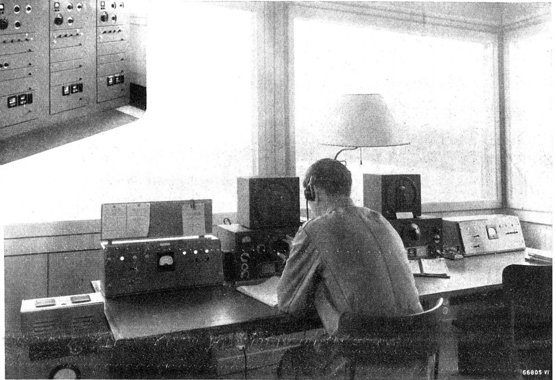
Zwei Arbeitsplätze im Peiler Genf mit je einem Fernbedienungsgerät zum 300-W-Sender
