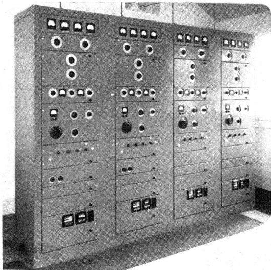
Vier zu einem Block vereinigte 300-W-Kurzwellensender in der Funkstation Avanche d. Flugplatzes Genf-Cointrin
