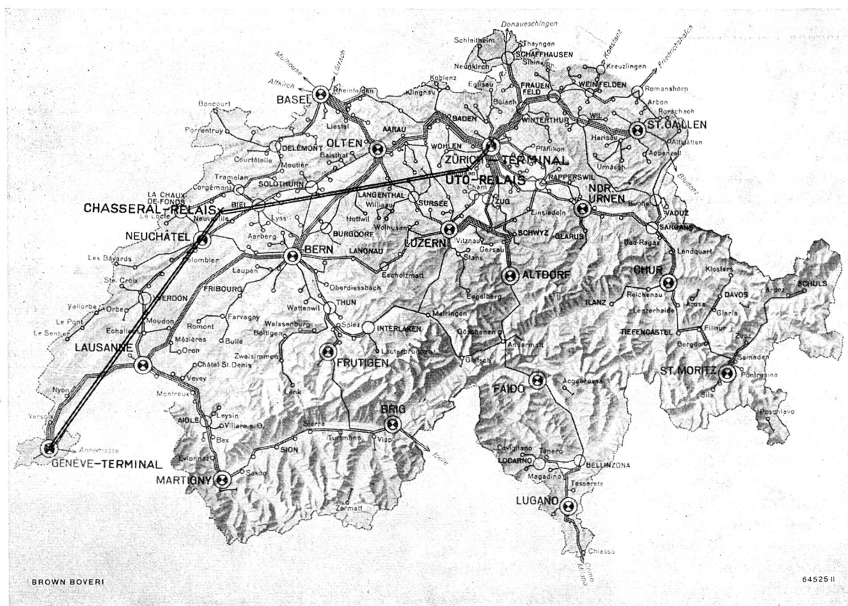
Das schweizerische Telephonkabelnetz mit eingezeichneter Mehrkanal-Richtstrahlanlage Zürich—Genf Die erste schweizerische Mehrkanal-Richtstrahlanlage Zürich—Genf mit je einer Relaisstation Uetliberg (Uto) und Chasseral ist mit Doppelstrich eingetragen. Die Länge der drei Teilstrecken beträgt zusammen zirka 241 km; sie steht seit Anfang Oktober 1947 als Versuchsanlage im praktischen Telephonbetrieb der PTT.
