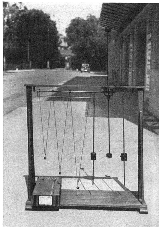
Pendelmodell in Ruhe.
