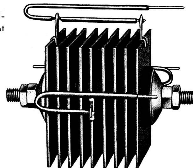
Kupferoxydul- Gleichrichterelement
