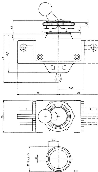
Abmessungen des Kippschalters
