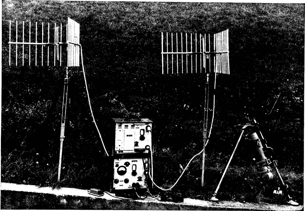
Vollständige Richtstrahlstation mit Frequenzmodulation für Betrieb im Gegensprechverkehr über eine Distanz bis zu 200 km Links: Sendeantenne, rechts: Empfangsantenne, Mitte: Apparatkasten, rechts aussen: Tretgenerator
