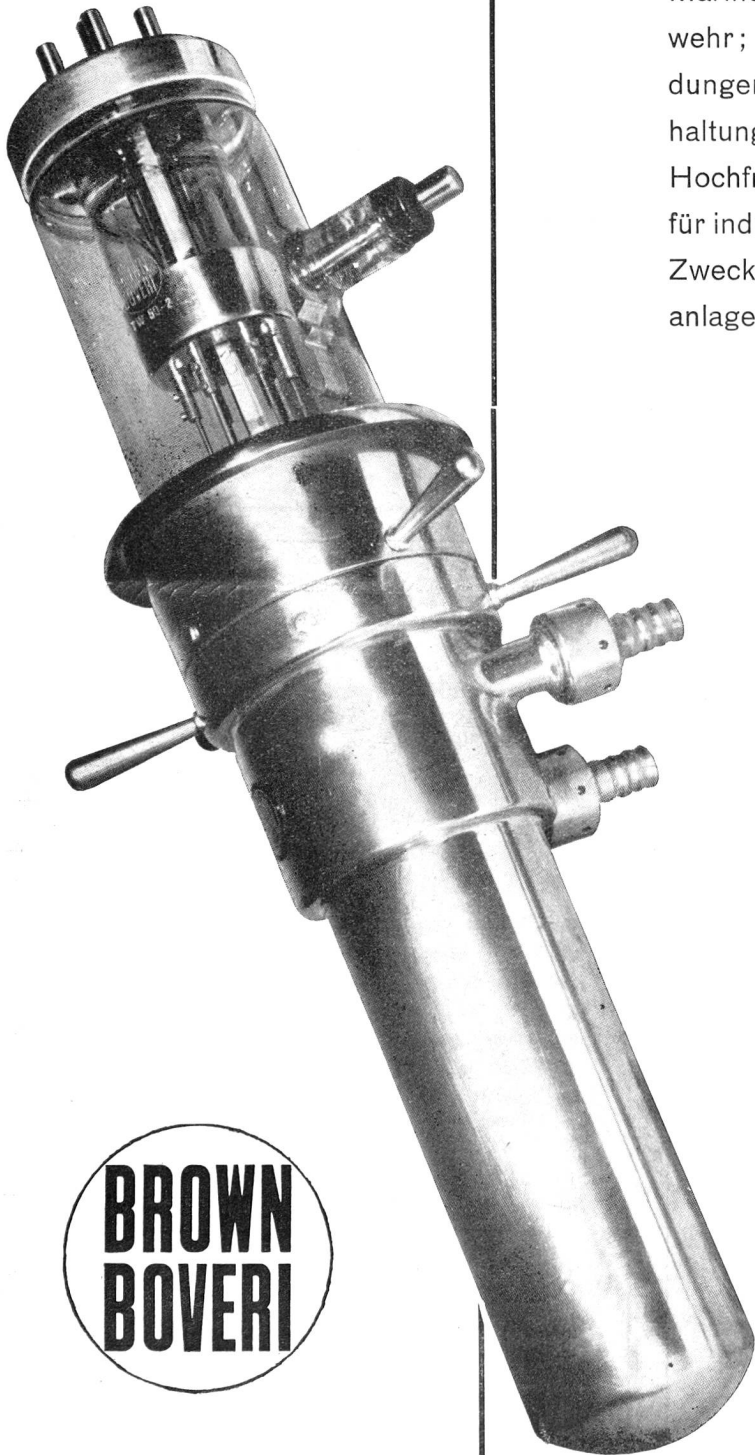
Wassergekühlte Senderöhre für mittlere und kurze Wellen
