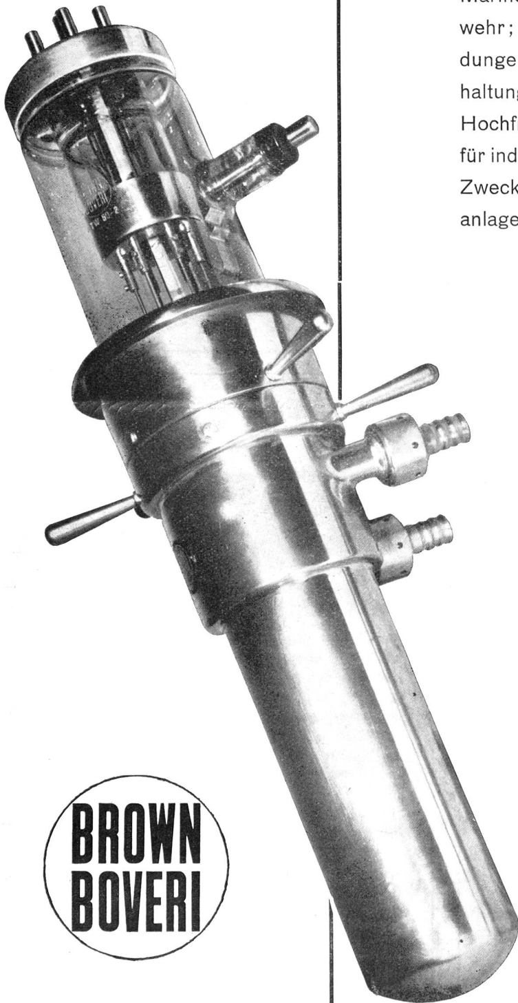
Wassergekühlte Senderöhre für mittlere und kurze Wellen
