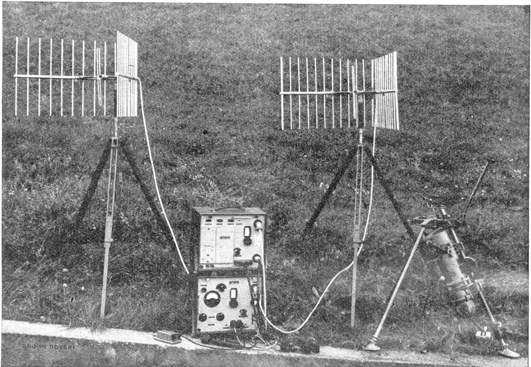
Vollständige Richtstrahlstation mit Frequenzmodulation für Betrieb im Gegenseprechverkehr über eine Distanz bis zu 200 km Links: Sendeantenne, rechts: Empfangsantenne, Mitte: Apparatekasten, rechts aussen: Treibgenerator
