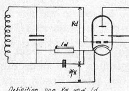
Definition von Kd und Id
