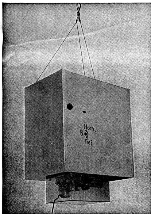
Radio-Sonde (Messgeräte und Sender)
