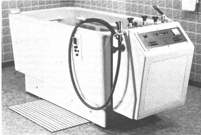
UKS-Fischer-Unterwassermassage-Anlage DE LUXE. Serienmäßige Ausführung mit Einrichtung für Unterwasser-Massagen, Vibrations-, Hitze- und Saugmassagen. Zusatzeinrichtung für elektro-galvanische Bäder.
