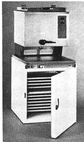
60 Lt. Fangoaufsetzgerät mit Auslauf montiert auf Fangowarmhalteschrank Typ 60. Dazwischen Querstromgebläse zur Kühlung der Fangopackungen.
