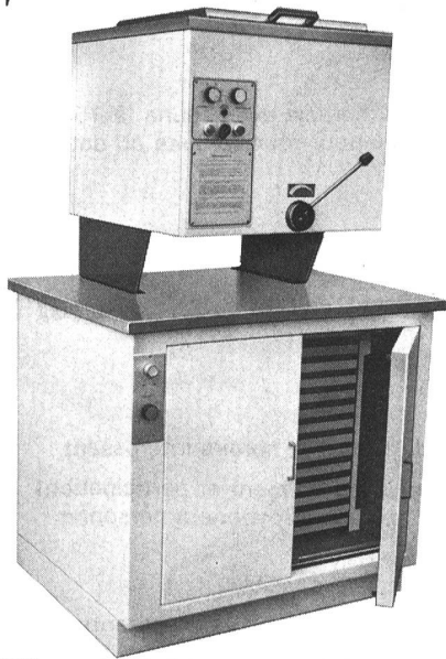
Rührwerk TA 60 (Liter) auf Warmhalte-schrank 5070, Edelstahlplatte 95x75.
