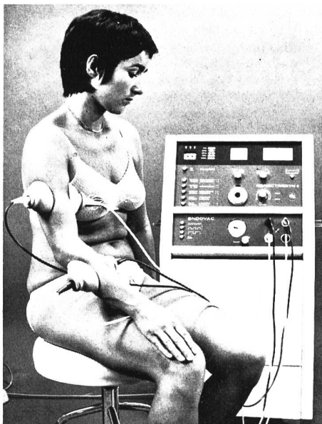
Das Standgerät Nemectrodyn 8
