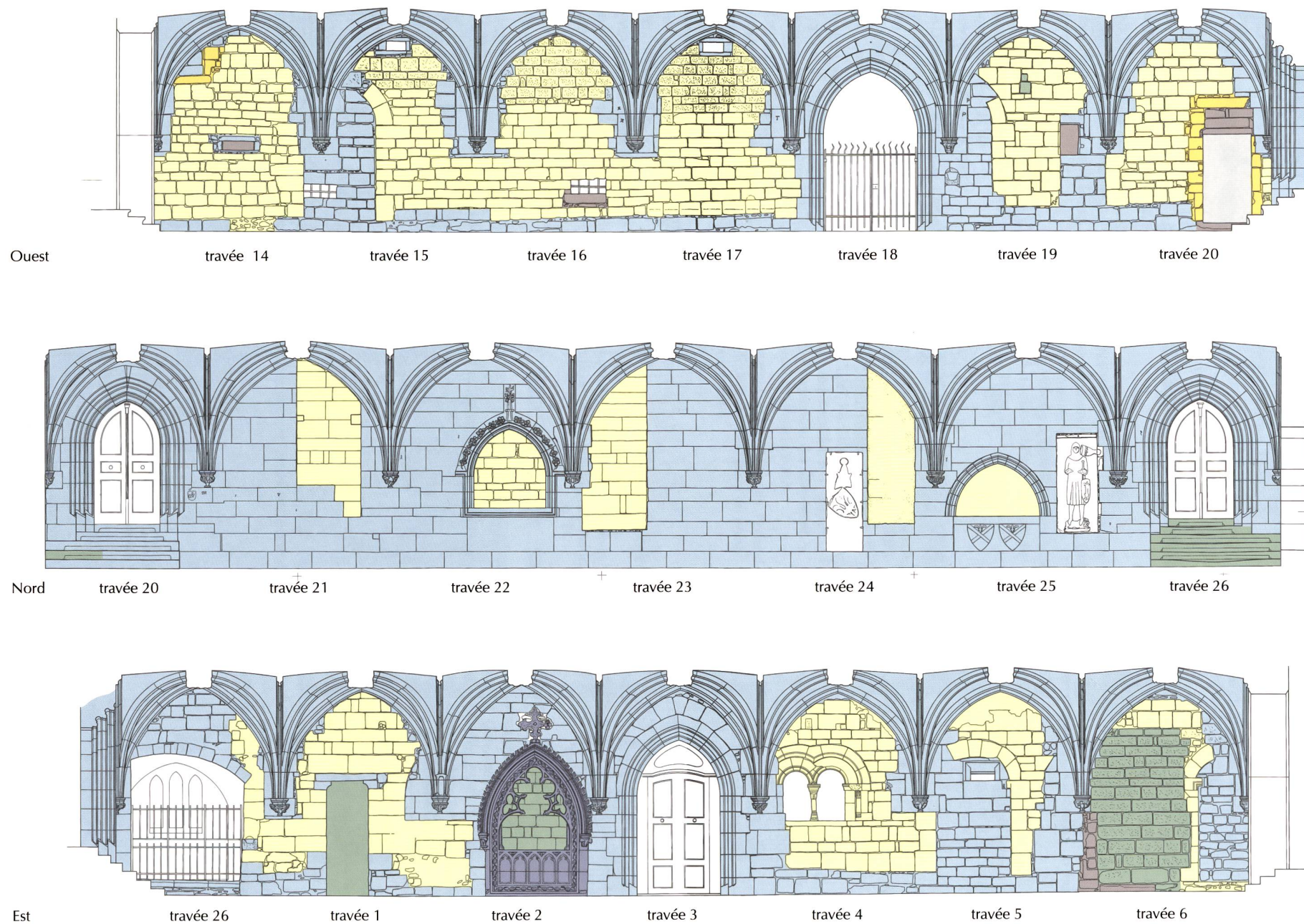
Fig. 133 Coupes longitudinales et élévations des murs des trois galeries du cloître. Abb. 133 Längsschnitte und Wandaufriß der drei Seiten des Kreuzgangs.
