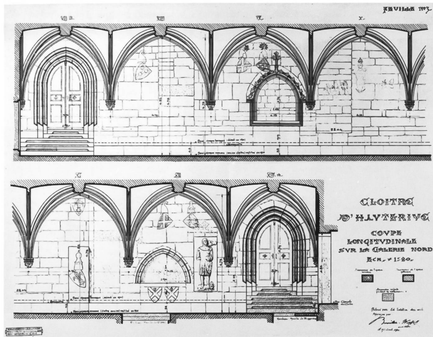
Fig. 131 Edmond Lateltin (1887-1952), «Cloître d'Hauterive, coupe longitudinale sur la galerie nord» (copie), 1911.
