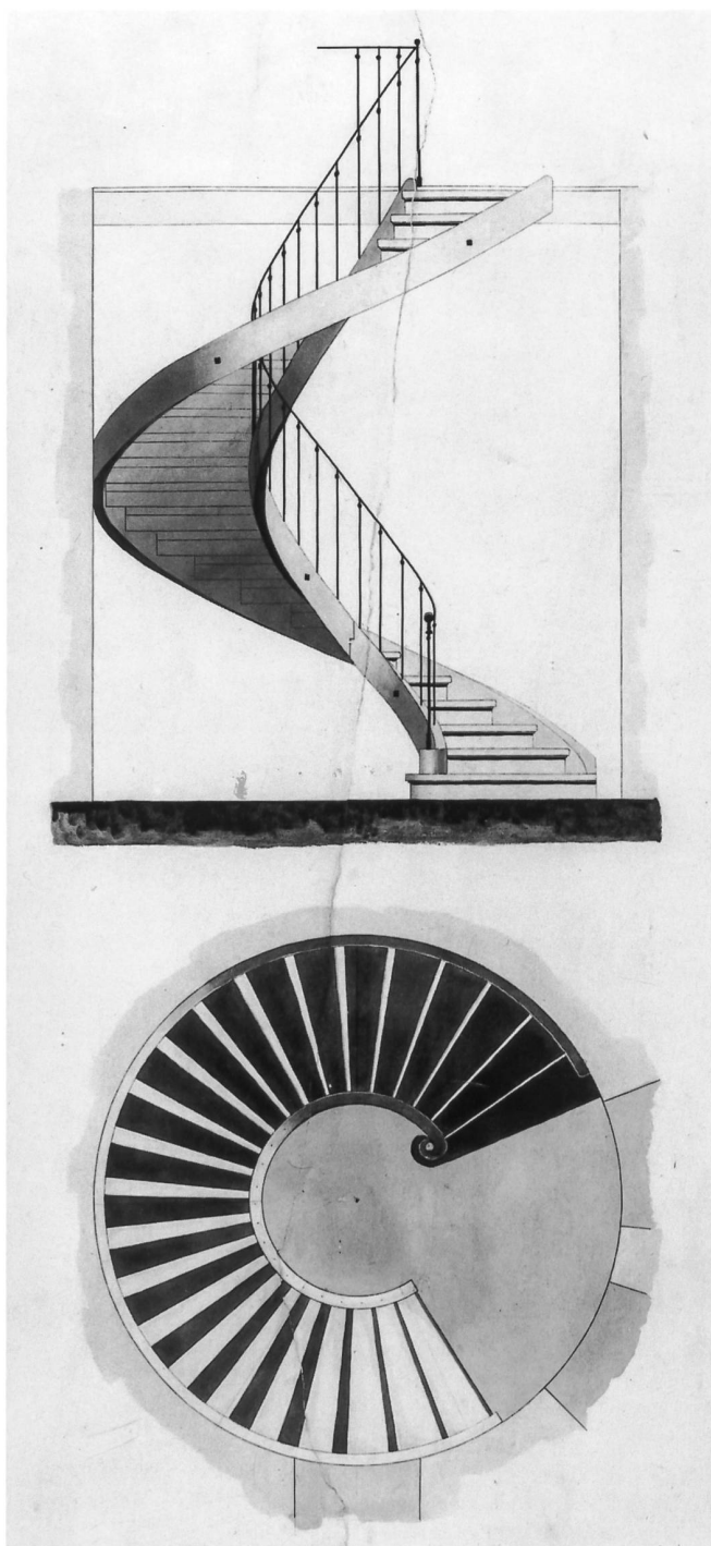
Fig. 114 Joseph-Emmanuel Hochstättler, architecte cantonal, Elévation et plan de l'escalier de la tour de l'horloge, 1851, plume et lavis sur papier, 52,6 x 66,3 cm (Archives de l'Etat de Fribourg). – Cet escalier a été conçu par Hochstättler pour desservir la caserne de gendarmes aménagée en 1851 au deuxième étage. Jusqu'alors, la tour était restée vide.
