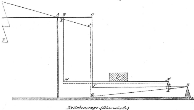
Brückenwage (Schematisch.)
