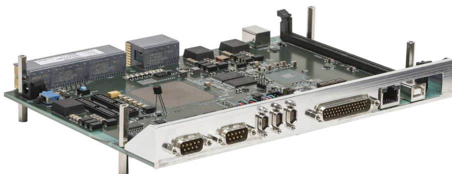
Abbildung 2: Der neue Lynx-Computer ist 250-mal leistungsfähiger als normale Bordcomputer. Die Entwicklung wurde mit Hilfe eines Vertrags aus dem Programm der Europäischen Weltraumorganisation für fortgeschrittene Forschung in Telekommunikationssystemen (ARTES) erreicht und bei RUAG Space in Göteborg, Schweden, durchgeführt.
